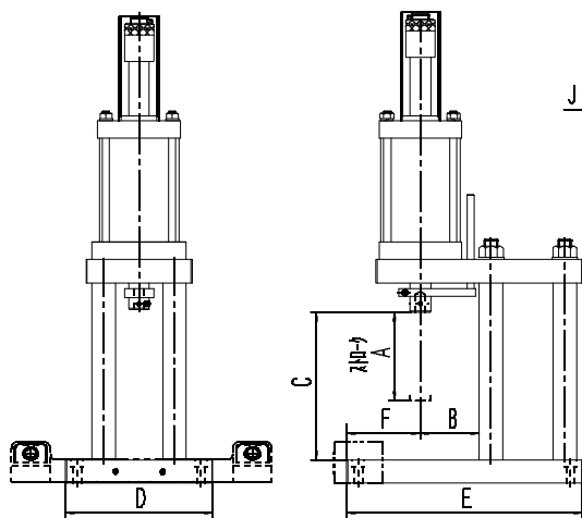
C型コラムプレス参考図
