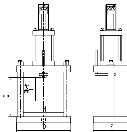
門型コラムプレス参考図
