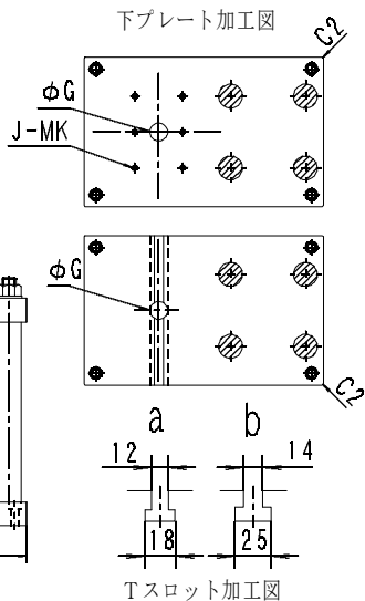
Tスロット加工図
